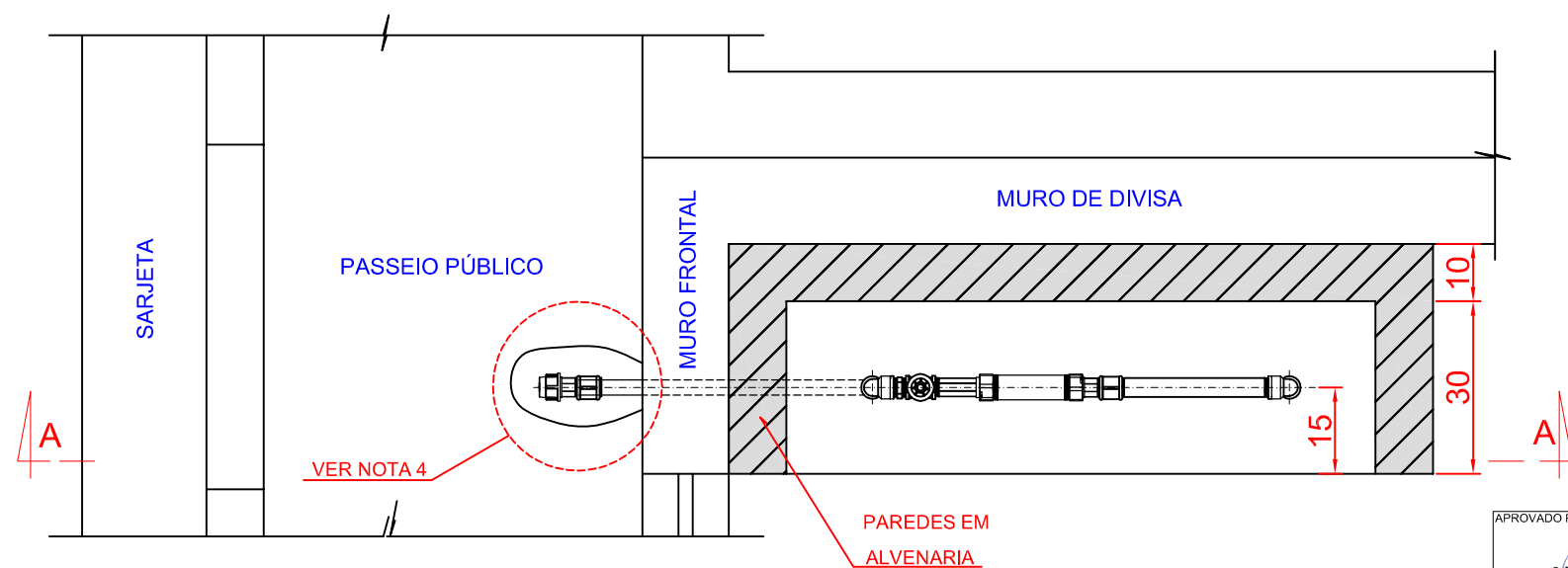
VISTA EM PLANTA
