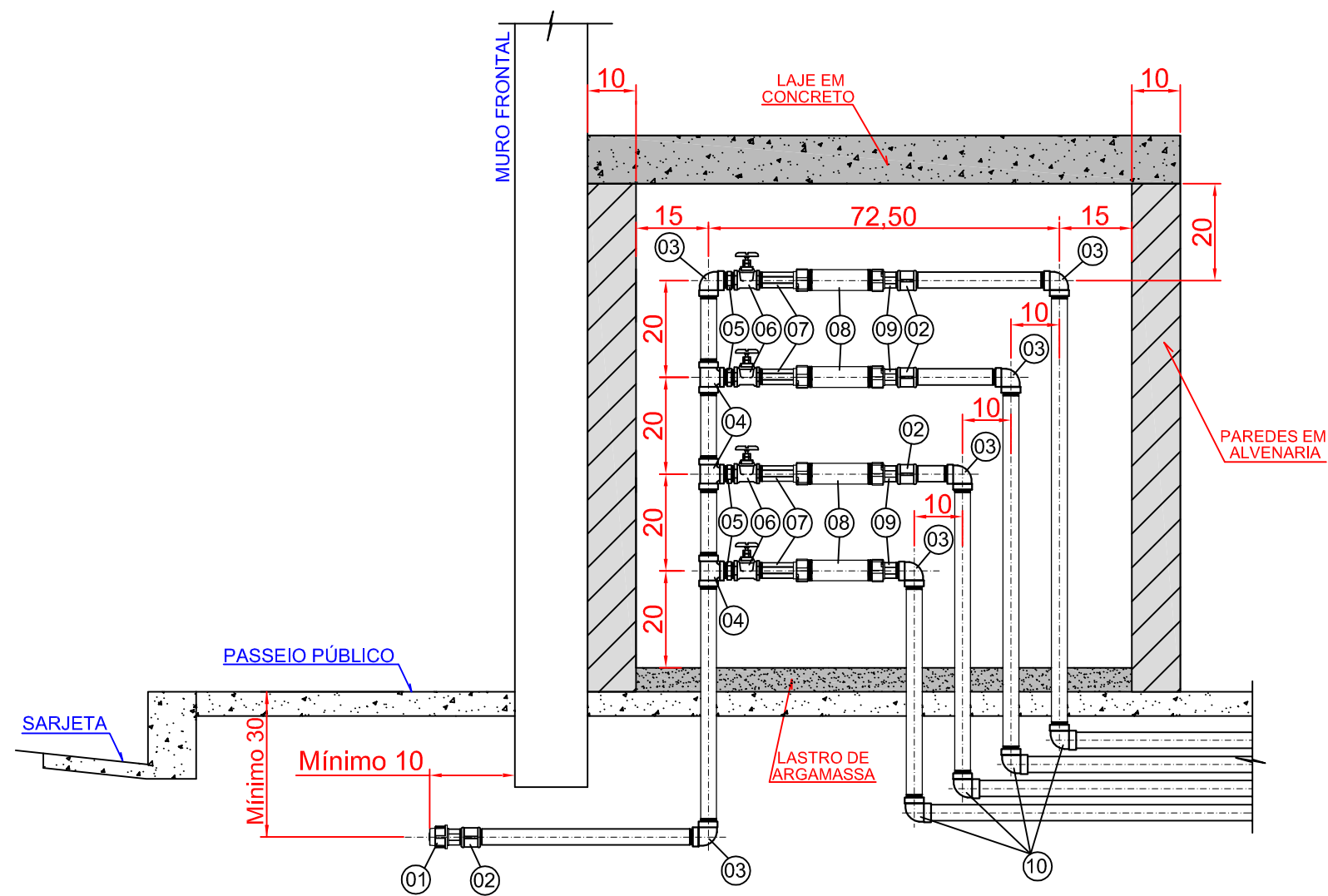
VISTA FRONTAL (CORTE "AA")
