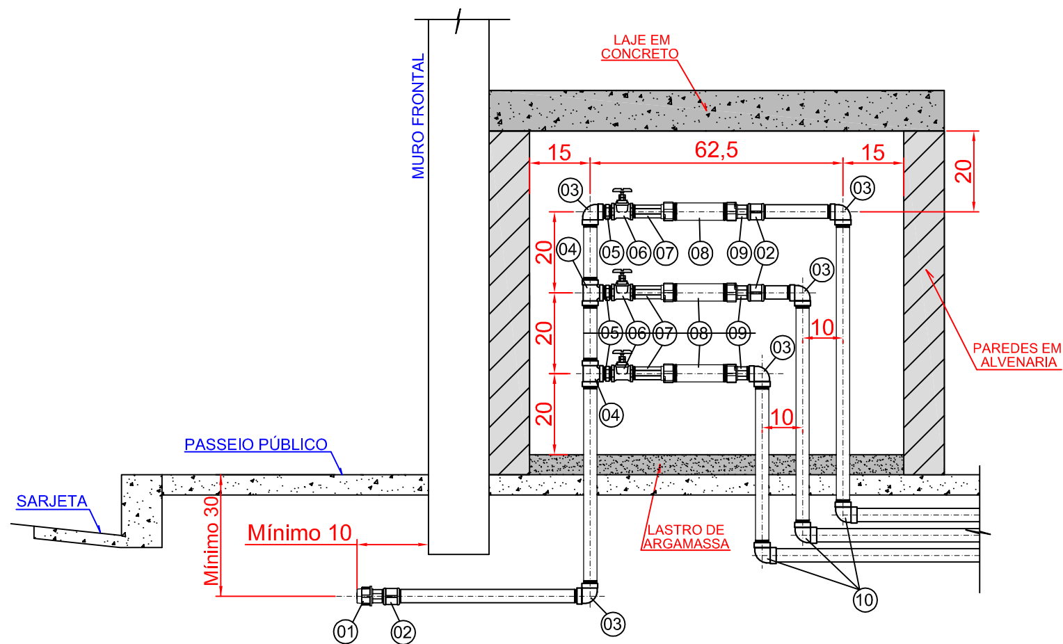
VISTA FRONTAL (CORTE "AA")
