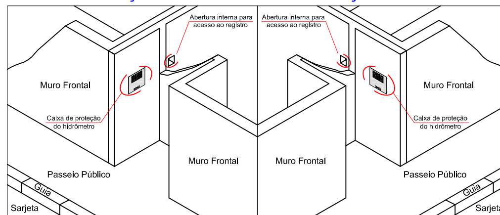
INSTALAÇÃO NO RECUE DE SERVIÇOS
