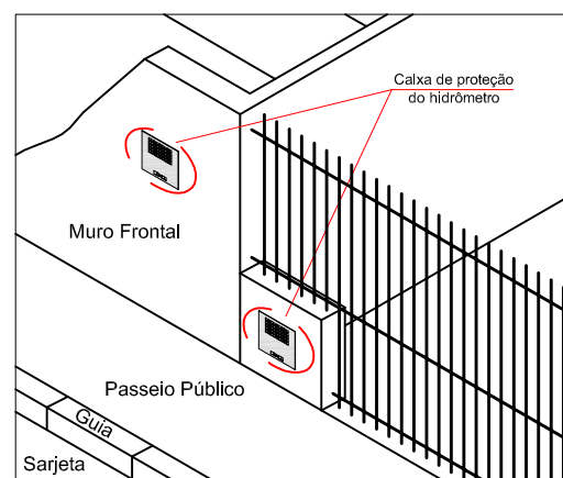
INSTALAÇÃO EM MURO FRONTAL
